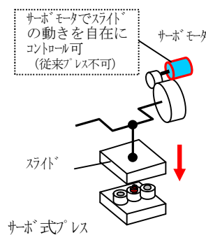
図. 鍛造用サーボ式プレス概略
