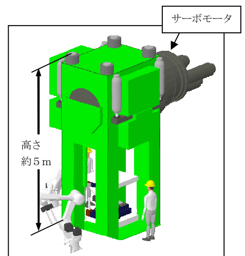
図. 鍛造用サーボ式プレス概略
